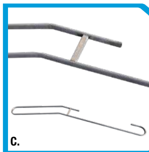
C. Tipologia corrimano per parete
