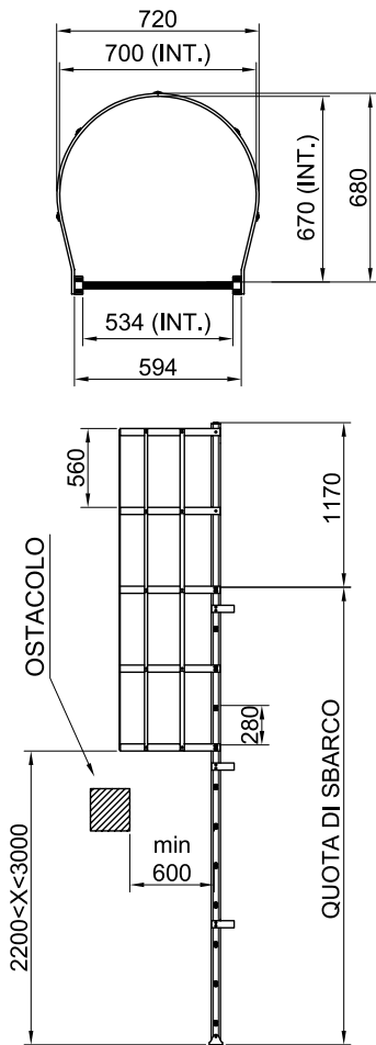
Scala tipo UNI EN ISO 14122-4
