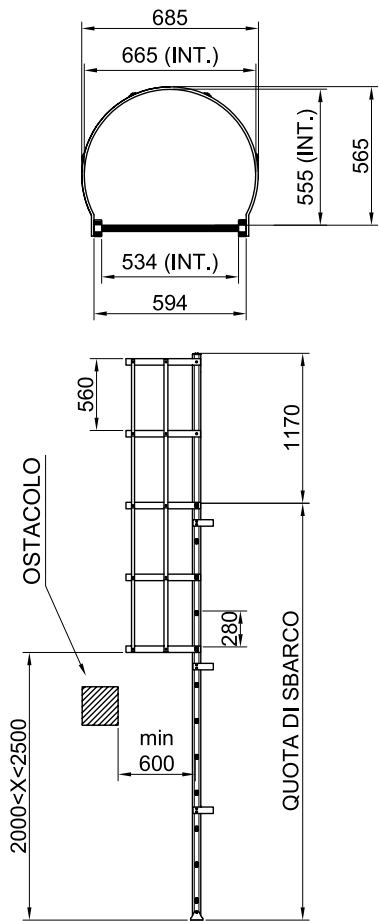
Scala tipo UNI 11962 - D.LGS. 81/2008
